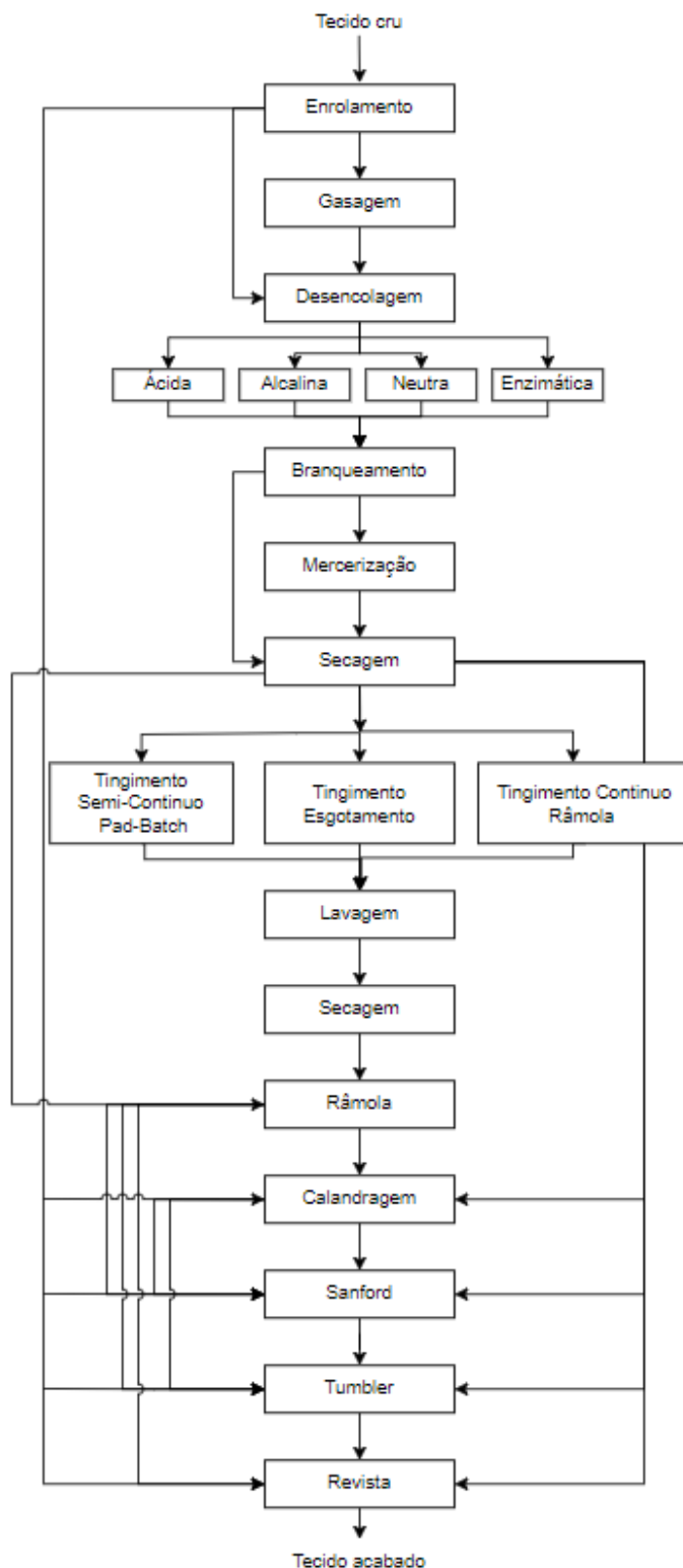
Figura 1 - Fluxograma Produtivo Vaz da Costa - Acabamentos.
